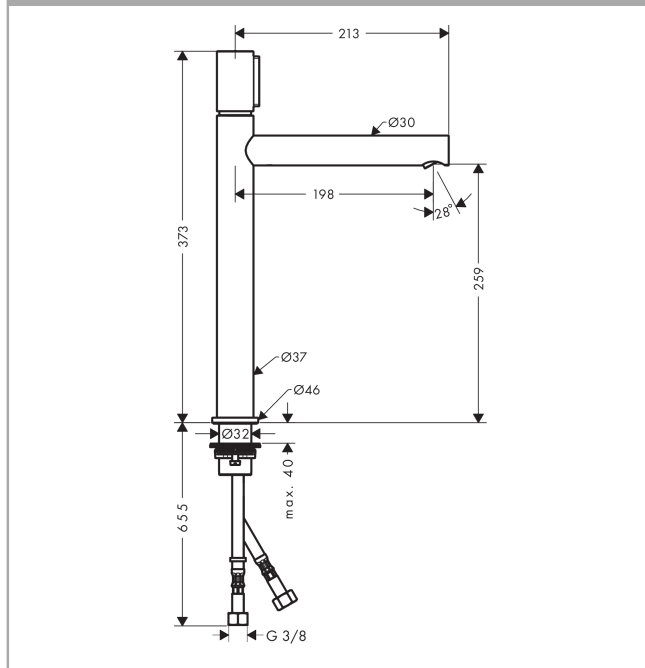
Maattekening
