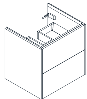
4.0227.2 - 8.6496.0 X. 595 mm Y. 595 mm Z. 490 mm
