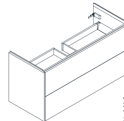
4.0237.2 - 8.6496.1 X. 790 mm Y. 595 mm Z. 490 mm
